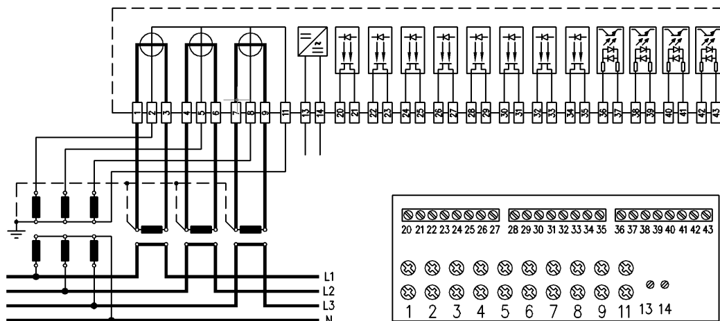
Figura 2 - Collegamento 3 sistemi 4 fili
