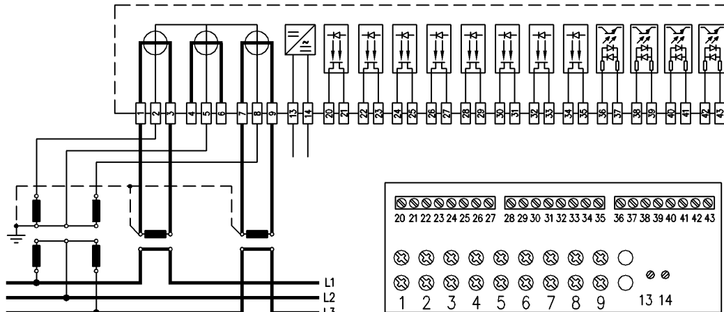
Figura 1 - Collegamento due sistemi 3 fili (Aaron)
